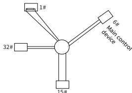
Рис. 7-3 Соединение звездой
